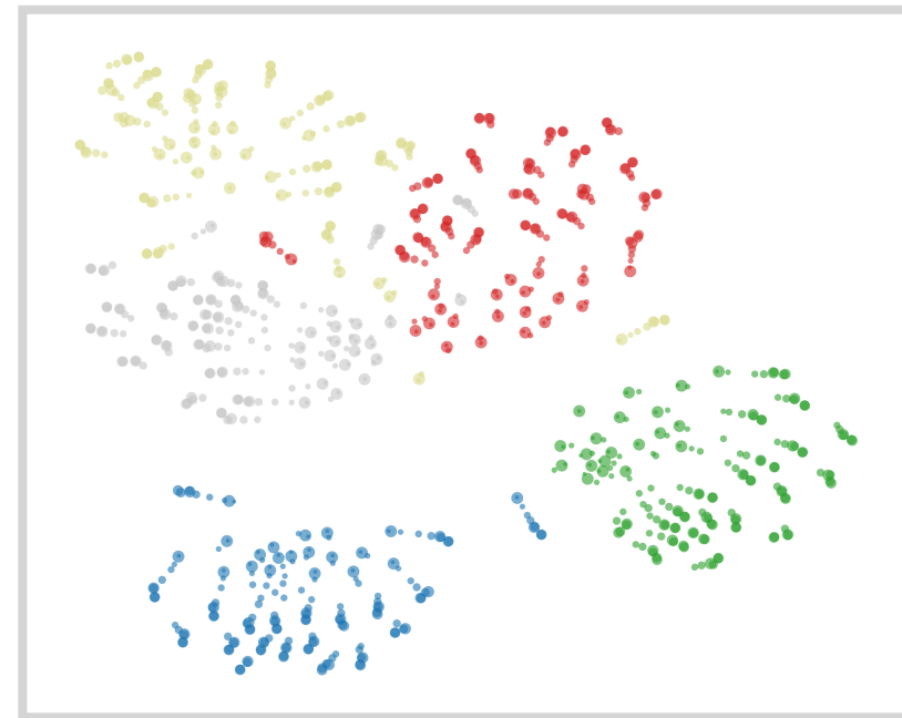
mLoRA
