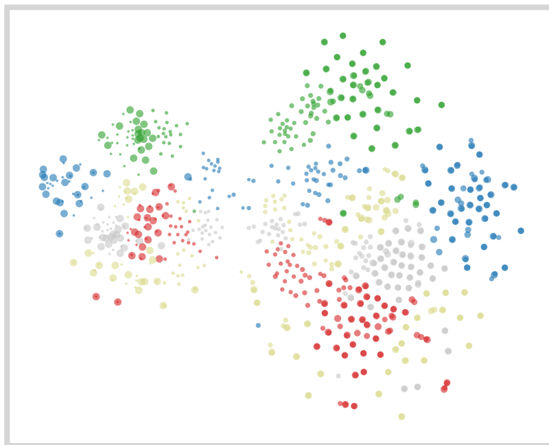
LoRA
