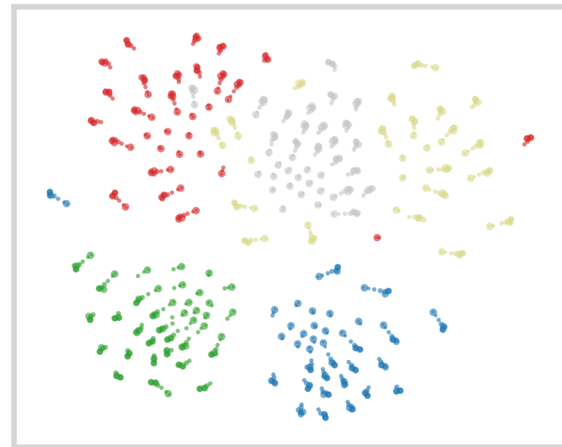
mLoRA-Asym
