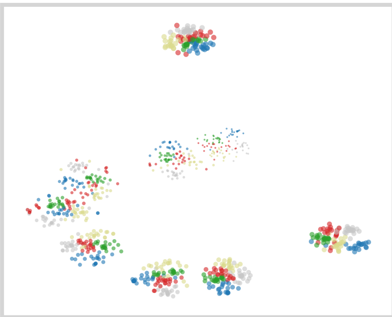
MLP-Asym
