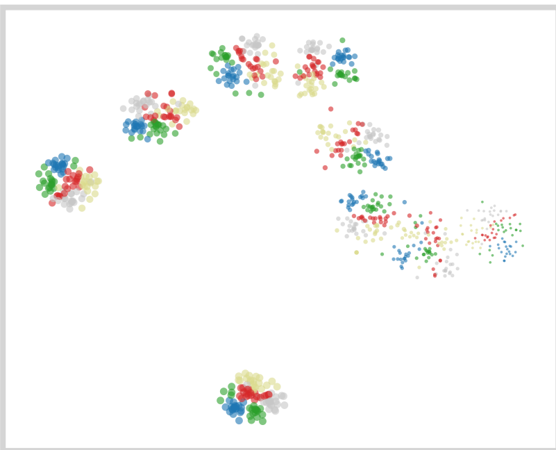
MLP
