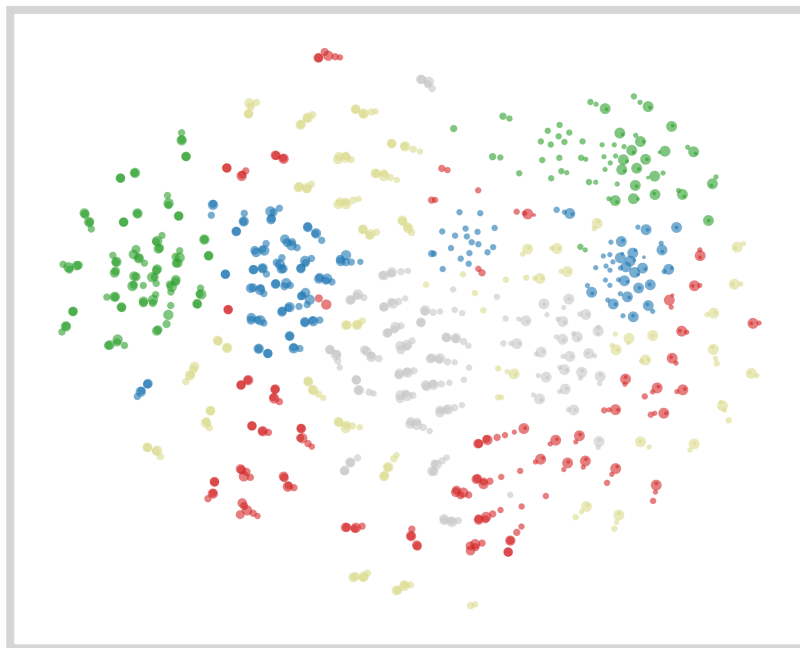
LoRA-Asym
